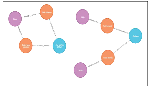
Gambar 12 Hasil query simpul Pembeli dan simpul UMKM yang dihubungkan dengan simpul Jual_produk
